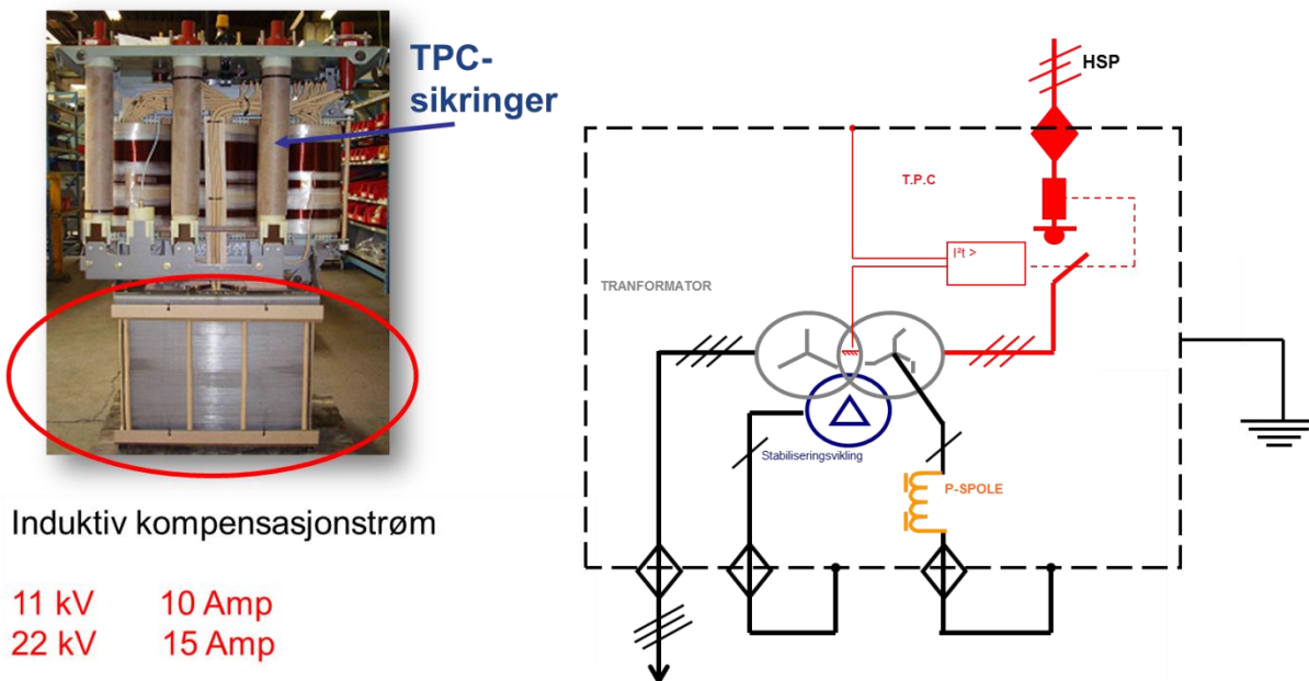
Koblingsgruppe ZN (d) Yn 11
